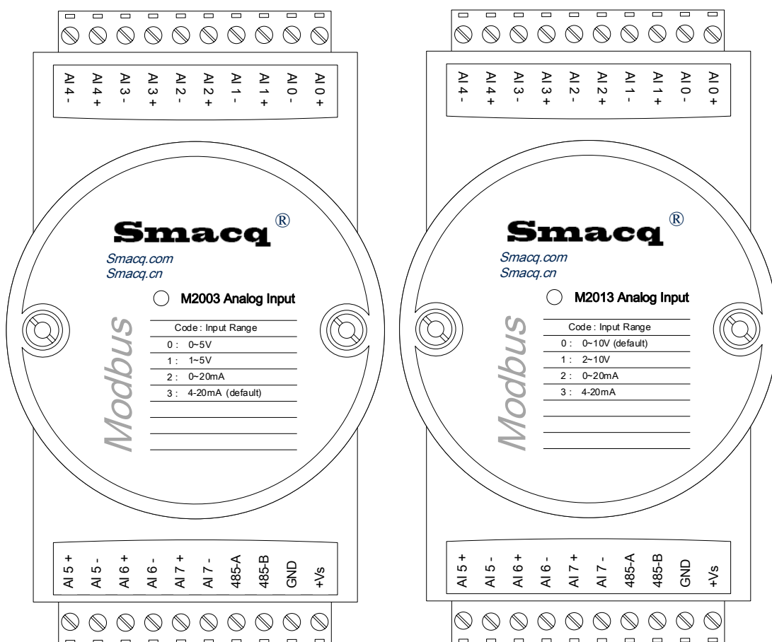
M2003 和 M2013 接线定义
