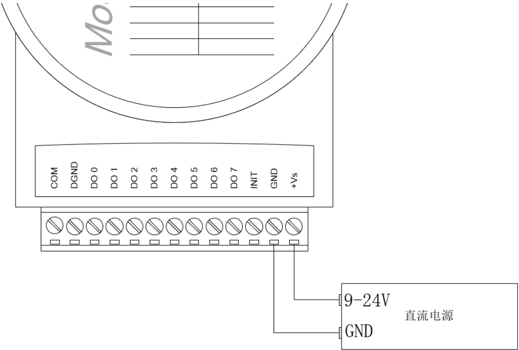
电源连接图
