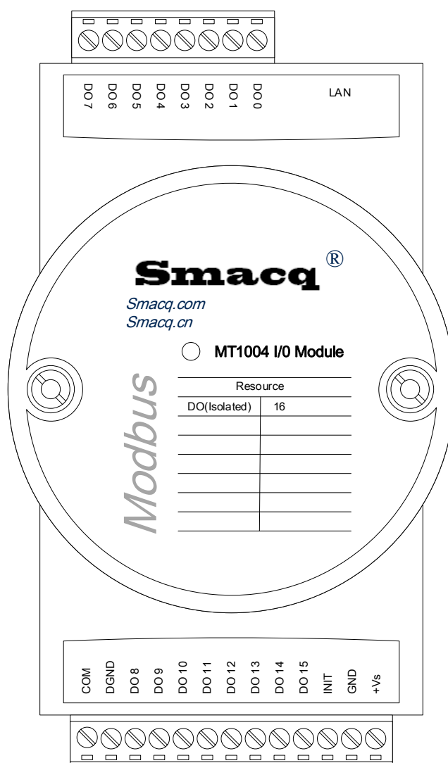
MT1004 接线定义
