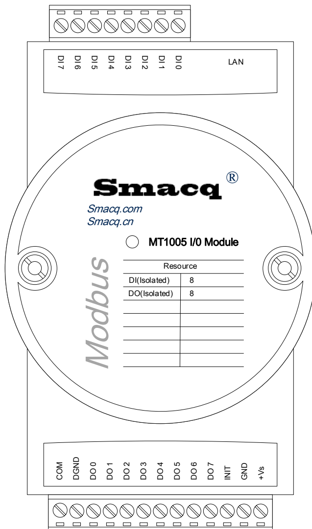
MT1005 接线定义
