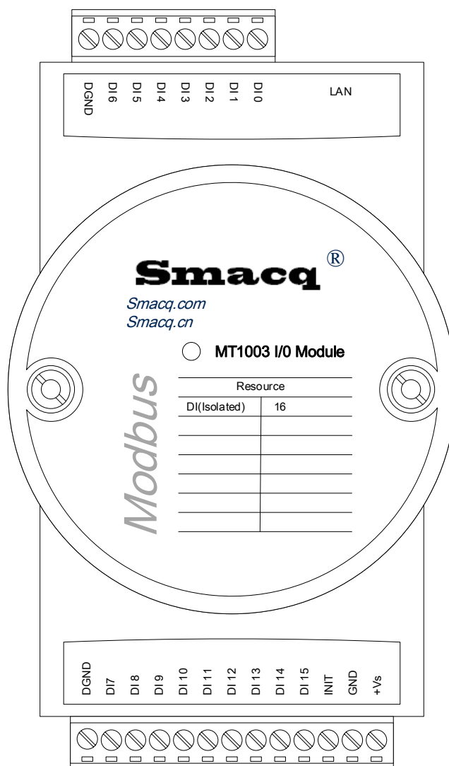
MT1003 接线定义
