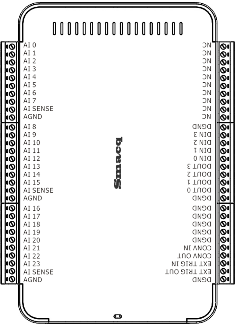
图 2.1、USB-3200 信号引脚分配图
