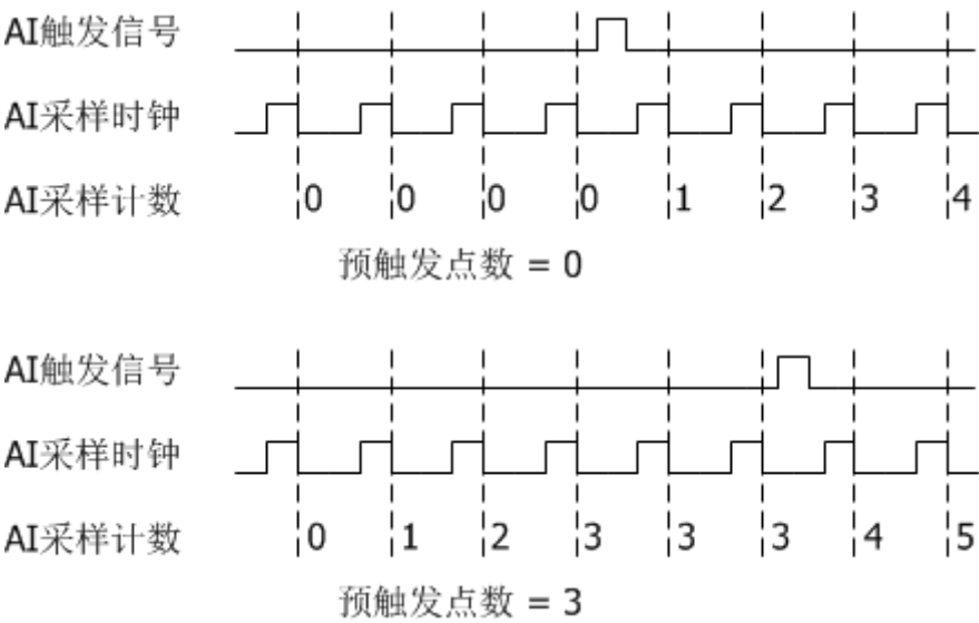
图 3.11、AI 预触发功能示意图
