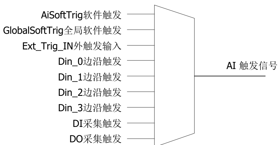
图 3.10、AI 触发选项示意图
