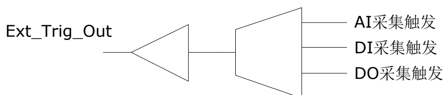
图 6.4、外触发输出电路示意图
