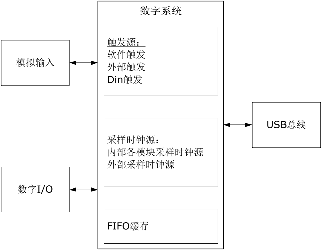
图 1.1、USB-3200 系列数据采集卡功能示意图
