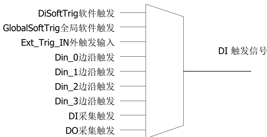
图 4.3、DI 触发选项示意图
