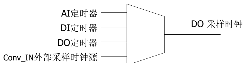
图 5.2、DO 采样时钟选项示意图
