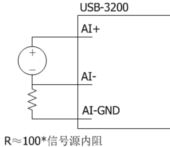
图 3.3、单个偏置电阻差分输入模式
