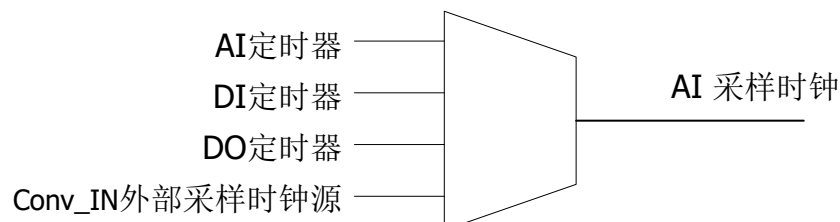
图 3.9、AI 采用时钟选项示意图
