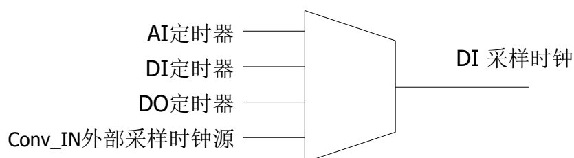
图 4.2、DI 采样时钟选项示意图
