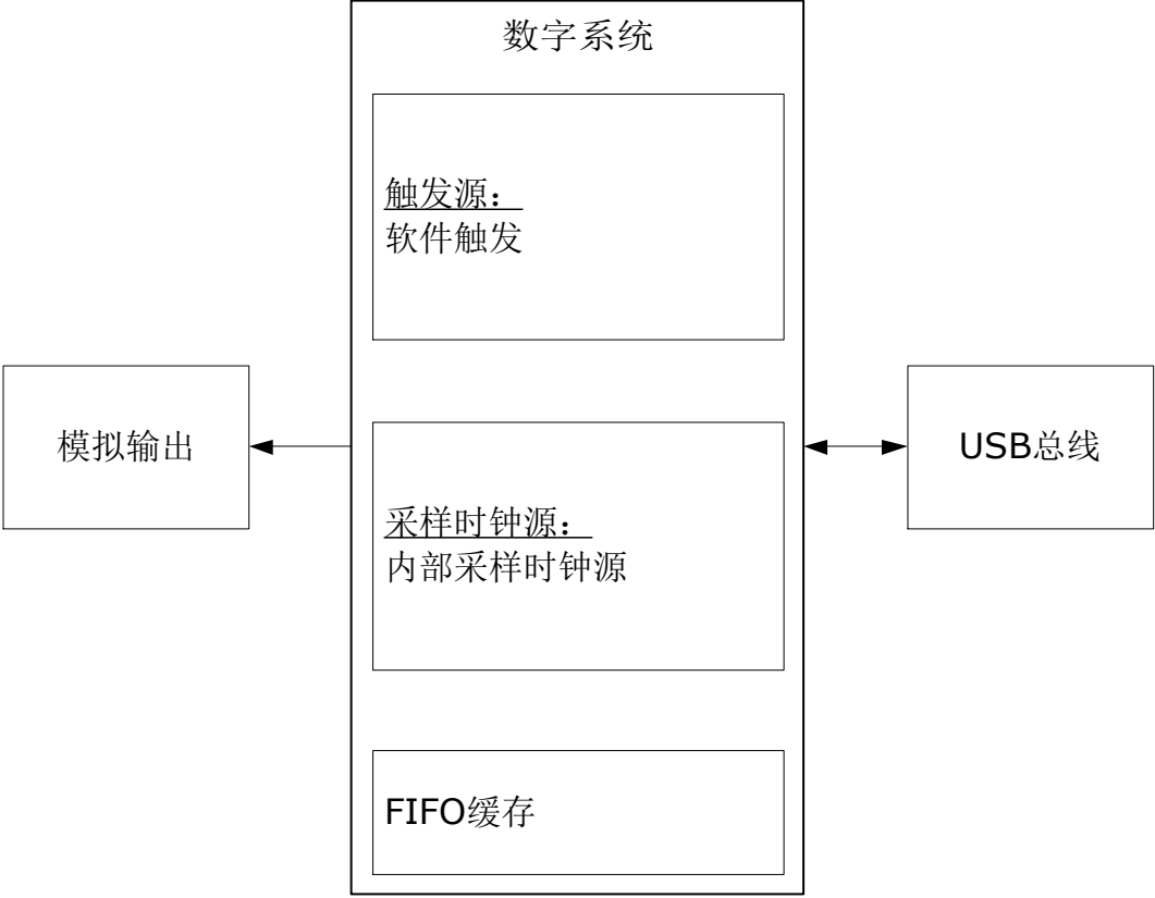
图 1.1、USB-3510 系列多通道模拟输出模块功能示意图
