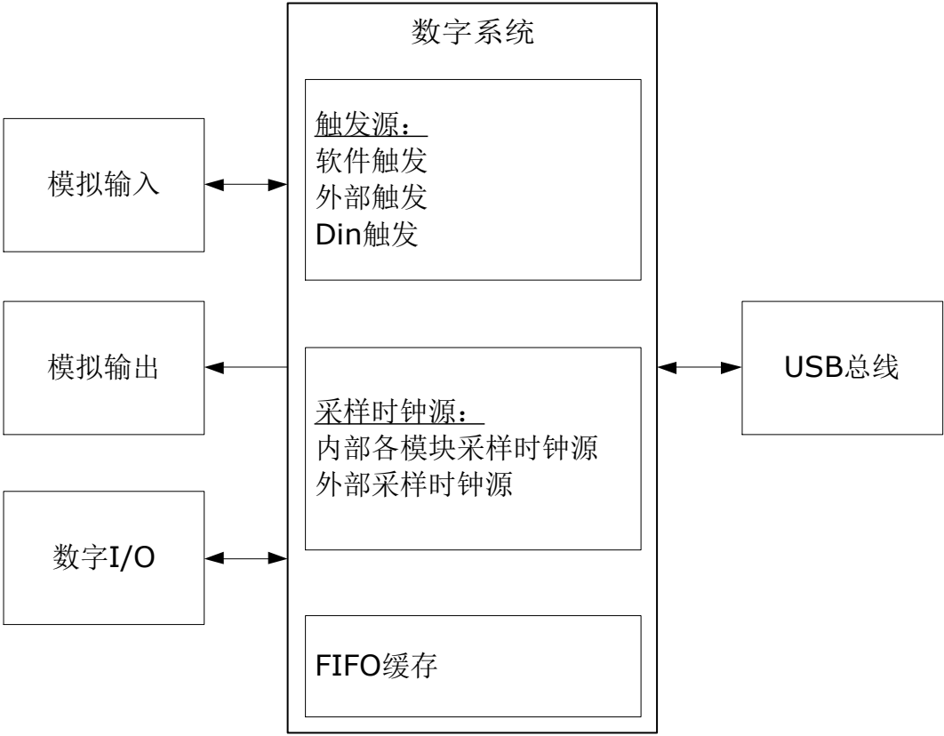
图 1.1、USB-5000C 系列数据采集卡功能示意图
