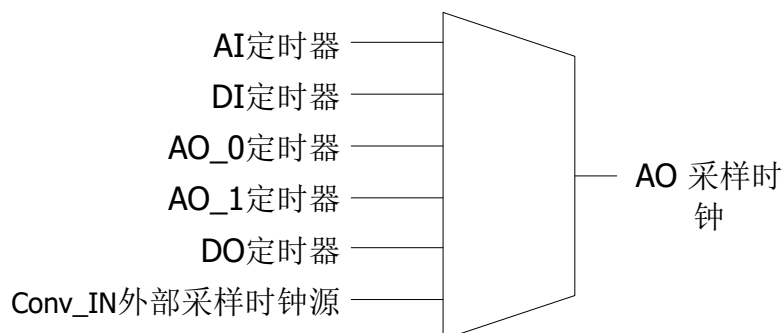
图 4.2、AO 输出采样时钟选项示意图
