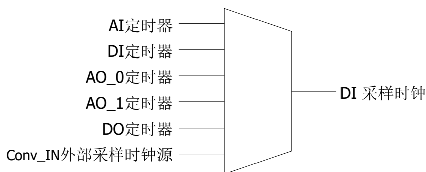
图 5.2、DI 采样时钟选项示意图
