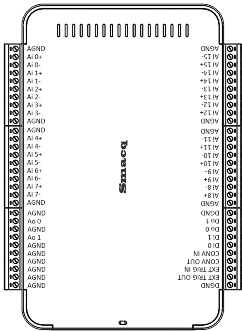
图 2.1、USB-5000C 信号引脚分配图
