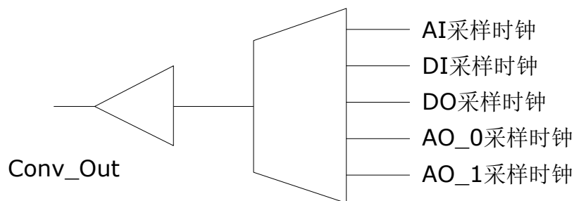
图 7.2、采样时钟输出电路示意图
