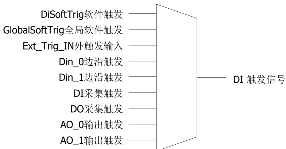
图 5.3、DI 触发选项示意图
